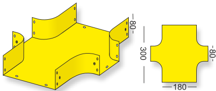
NAZWA ELEMENTU NR KATALOGOWY czwórnik koryt 18-08 EX-18-08
