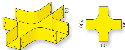
NAZWA ELEMENTU NR KATALOGOWY czwórnik koryt 08-08 EX-08-08
