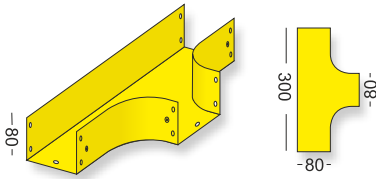
NAZWA ELEMENTU NR KATALOGOWY trójnik koryt 08-08 ET-08-08
